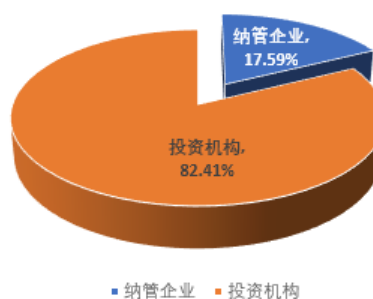
(右) 图 9 2018 上海碳市场各类型参与者交易量占比
