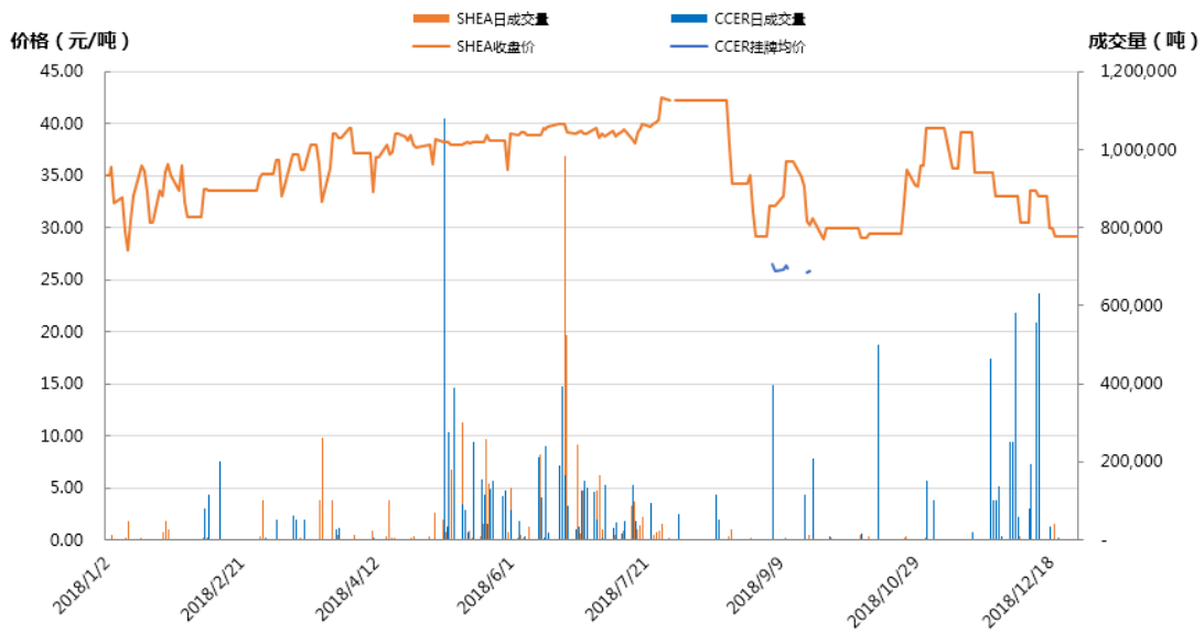
图 1 2018 年上海碳市场现货交易走势
