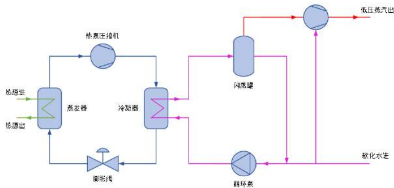
图2-6单级压缩+闪蒸+蒸汽压缩循环流程图
