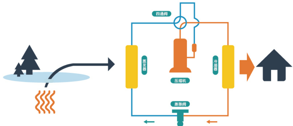
图2-4 土壤源热泵
